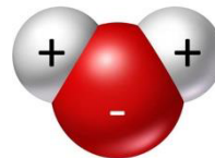
Abb.4 Wassermolekül
